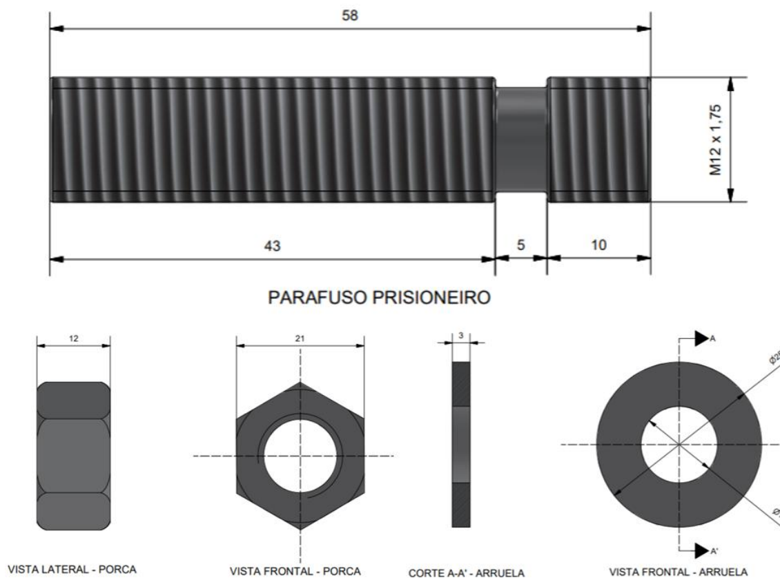
Figura 1 - Parafuso prisoneiro M12
